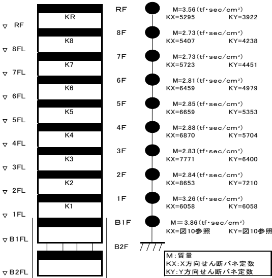
図 -1 建物モデル
