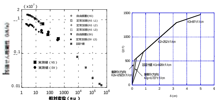
図-5. 等価剛性と相対変位
