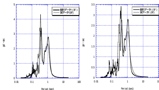
図-7. 修正復元力特性による解析結果と観測結果の比較 (左：X方向，右：Y方向)
