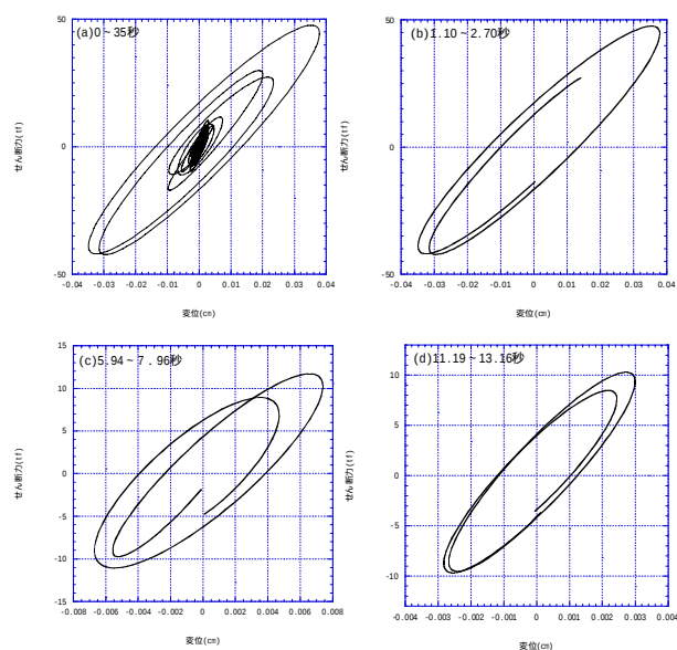
図-4. 地震観測記録から得られた免震層の復元力特性
