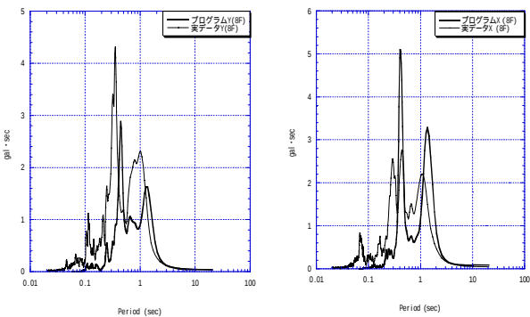
図 -2. 解析結果と観測結果の比較
