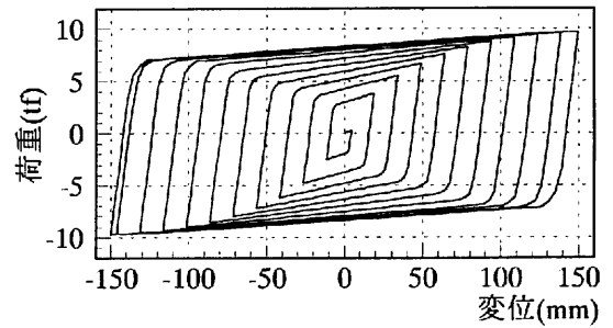
図3 提案する鉛ダンパーの復元力モデルによるU180 鉛ダンパーの漸増変位振幅解析結果
