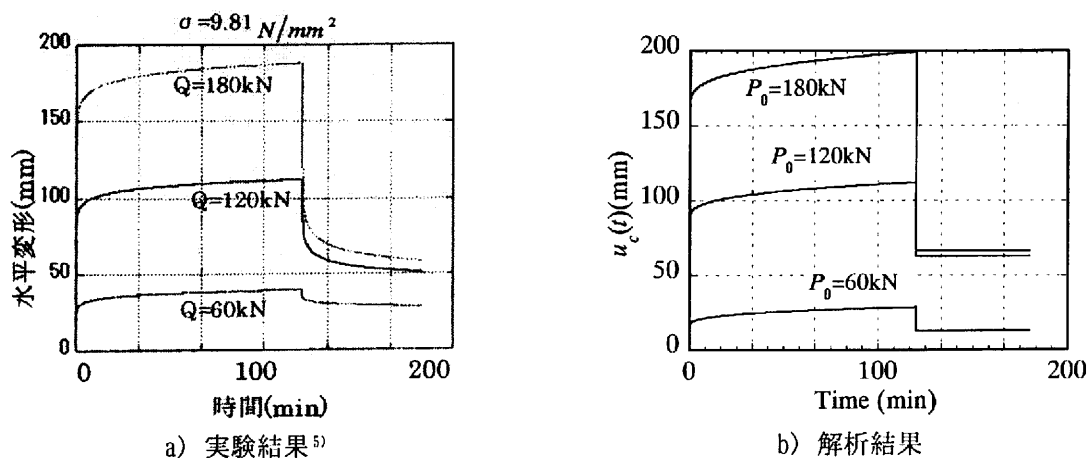
図8 一定水平加力試験結果と解析結果の比較
