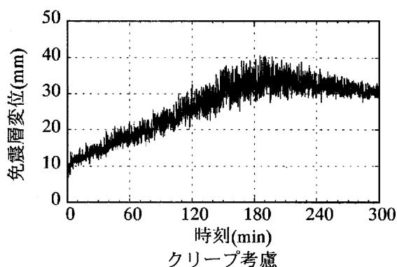
図11 免震層の変位時刻歴波形
