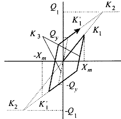
図2 鉛ダンパーの復元力モデル
