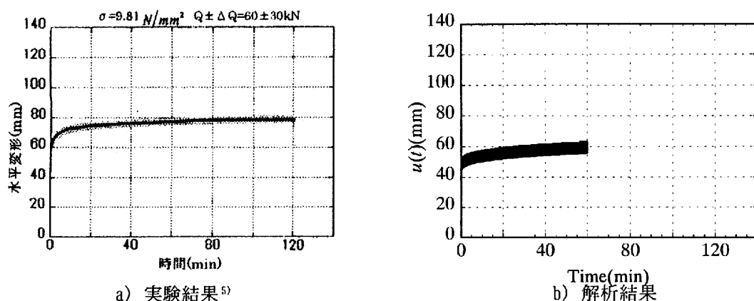
図9 一定荷重(60kN)+正弦波荷重( \pm 30 kN)試験による時間-変形関係の実験結果と解析結果の比較
