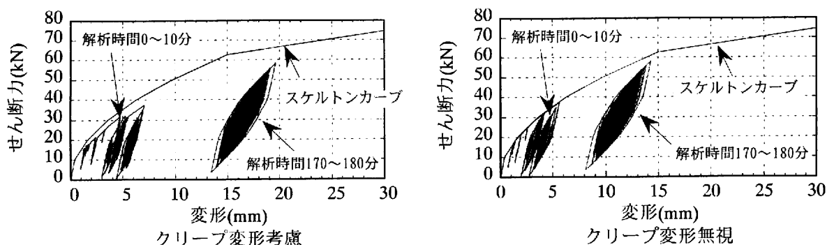
図 13 LRB 積層ゴム (縮尺試験体) のせん断力-変形関係
