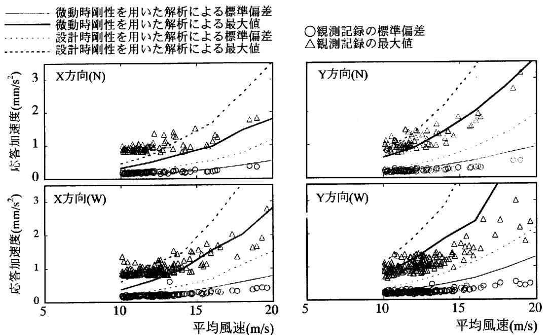
図6 風観測結果 6) と風応答解析結果の比較
