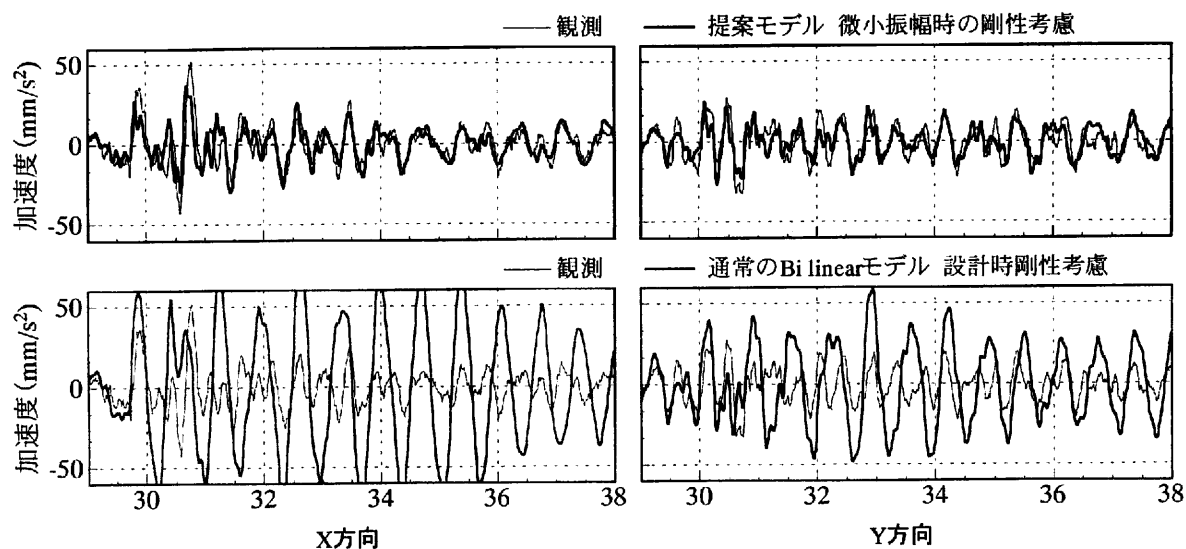
図5 地震観測結果 6) と地震応答解析結果の比較
