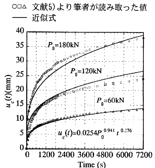
図 7 一定水平力加力実験に基づくクリープ変形の性状
