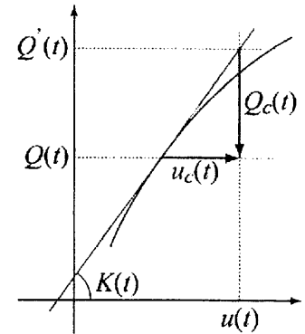
図4 内力とクリープ変形の関係
