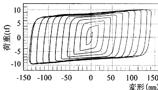
図1 U180 鉛ダンパーの漸増変位振幅実験結果 8)
