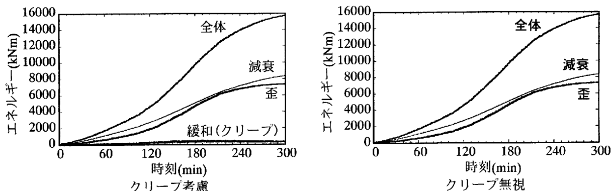
図 12 エネルギーの時刻歴波形
