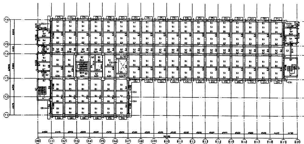
図—1 基準階伏図
