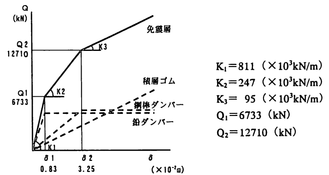
図一 4 免震層の復元力特性
