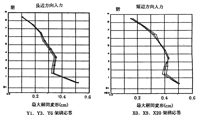
図-6 重心位置および最外周架構変形 （レベル2、ねじれ考慮 最大層間変形）
