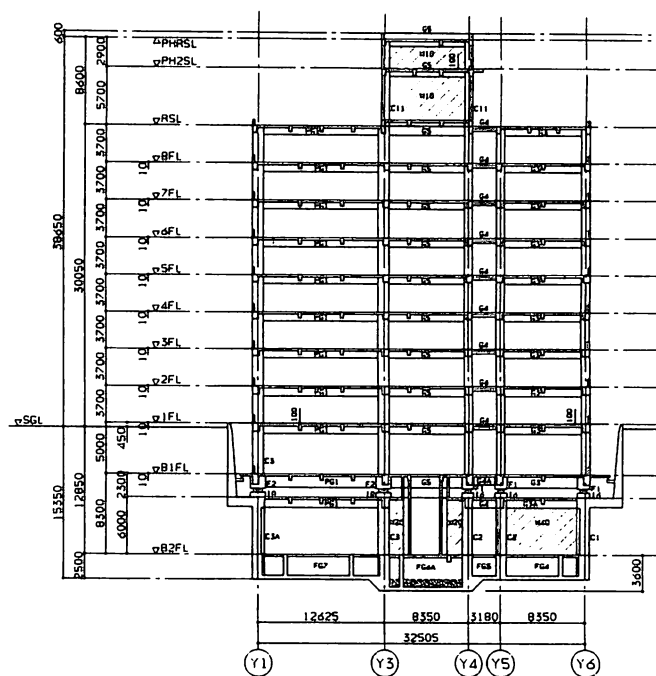
図—2 軸組図
