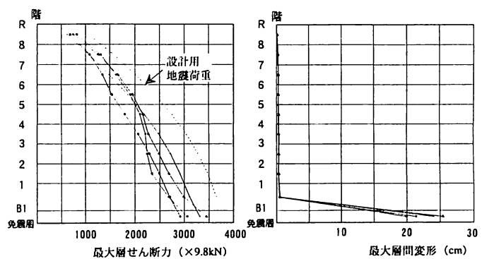
図-5 レベル2地震動時応答解析結果
