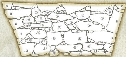
竹田城跡の石積の構造
