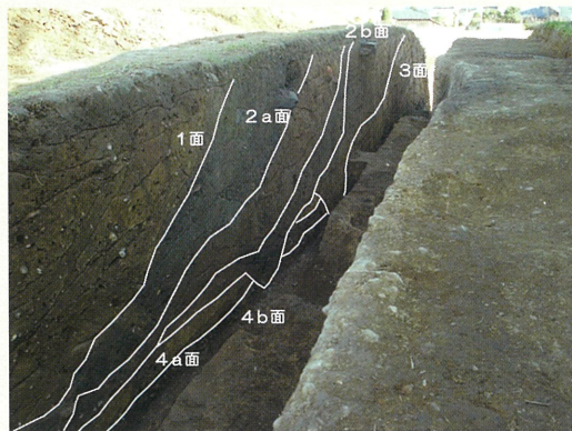
土塁跡断面
