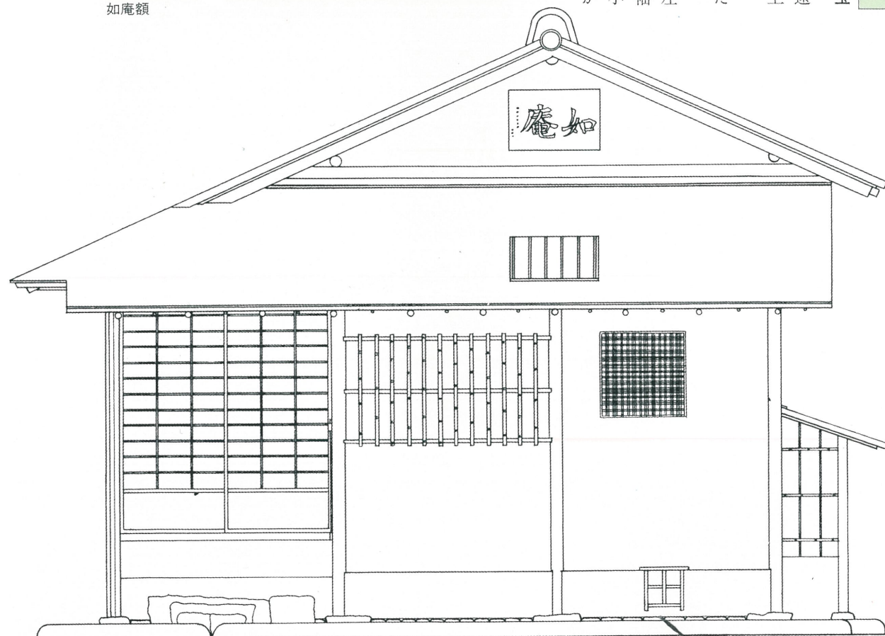
如庵立面図(正面)
