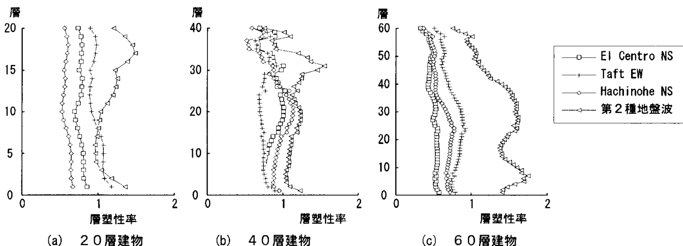
図-15 最大応答層塑性率
