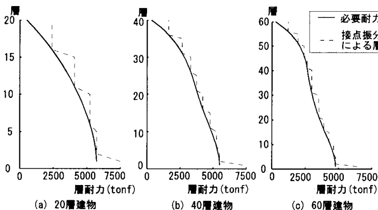
図-12 設定した建物層耐力
