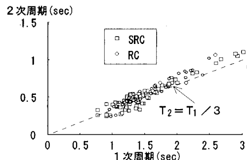
(b) 1次周期と2次周期
