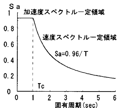
(a) 加速度応答スペクトル
