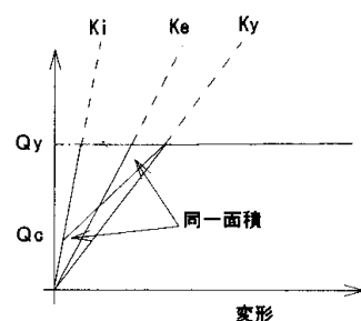
図-2 等価バイリニアモデル
