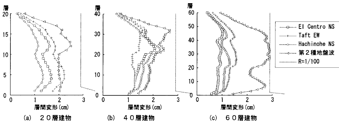
図-14 最大応答層間変形
