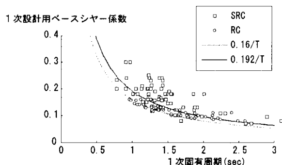
(a) 精算による1次固有周期
