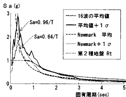
(a) 実地震動の加速度応答スペクトルとの比較
