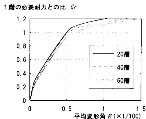
図-13 設定した建物の1階耐力比-平均変形角関係
