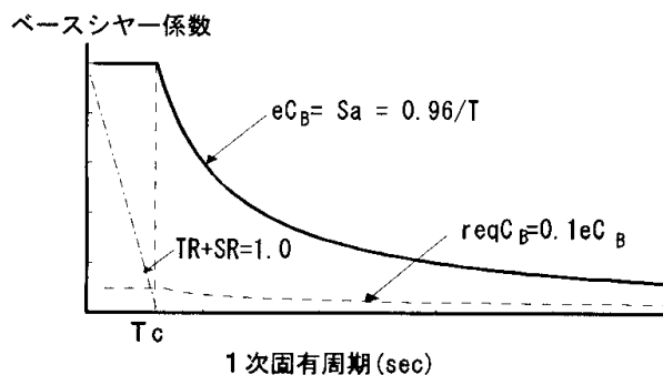
図-7 ベースシヤ-係数スペクトル
