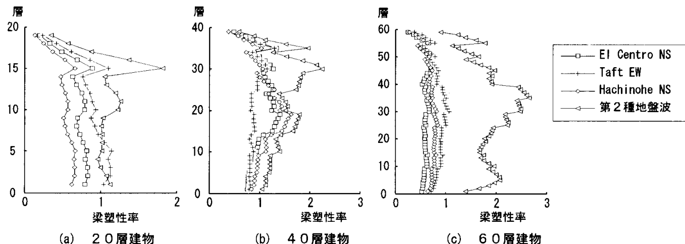
図-16 梁部材の最大塑性率分布
