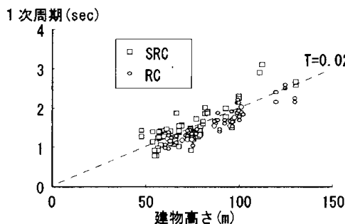
(a) 建物軒高さと1次周期
