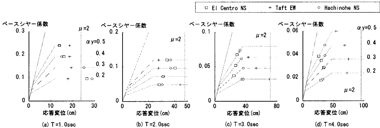
図-11 1質点系の地震応答解析結果
