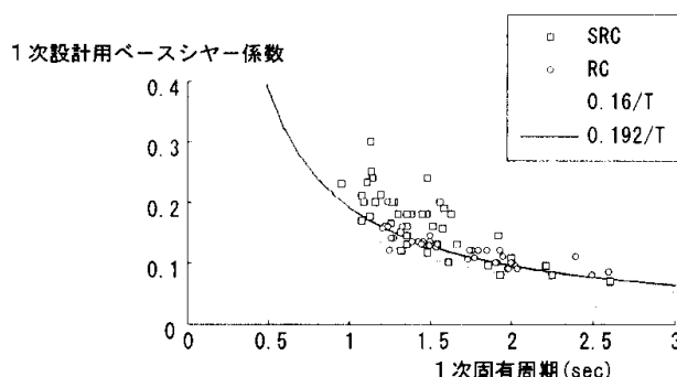
(b) 略算(T=0.02h)による1次固有周期
