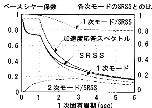
(b) ベースシヤ-係数
