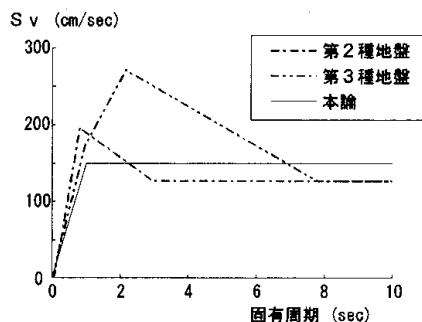
(b) 文献16)による設計用速度応答スペクトルとの比較
